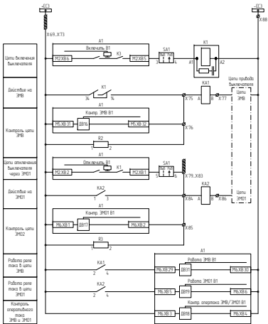
Цепи ЗМВ и ЗМО1
